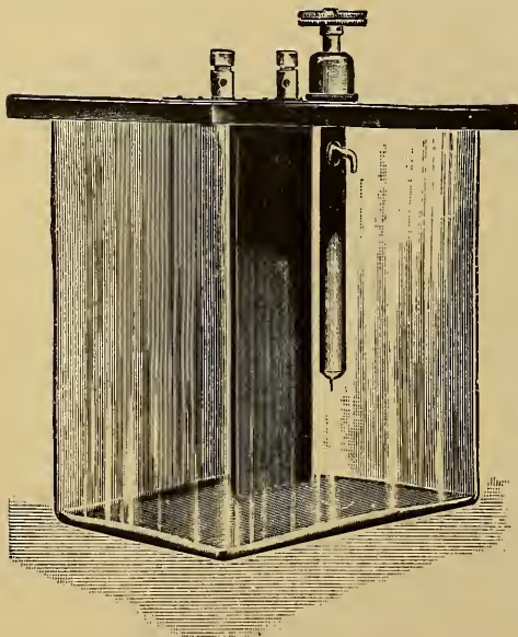
Fig. 38.—Wehnelt Interrupter. (Williams.)
