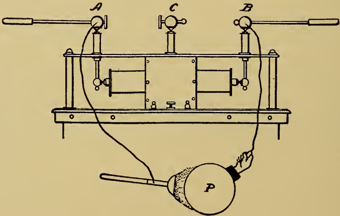
FIG. 117.—Tesla-Effluve.
