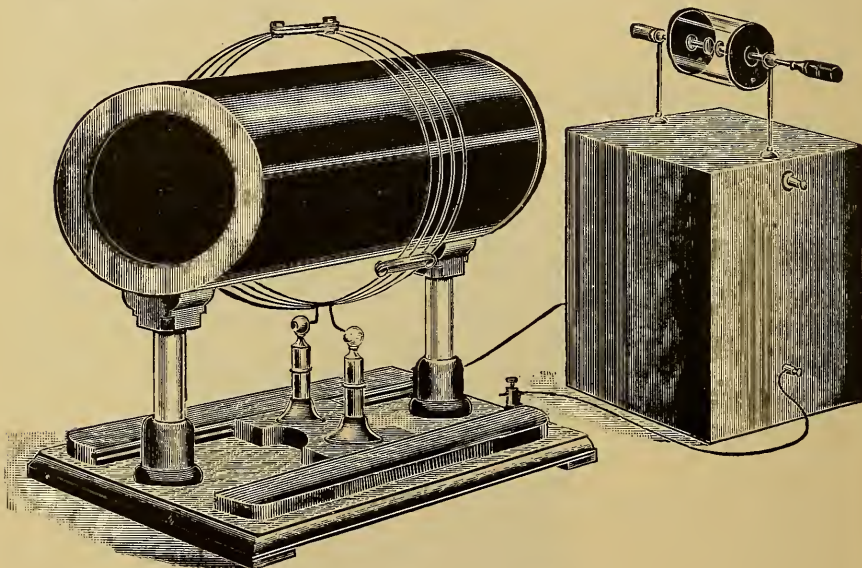
FIG. 45.— Gaiffe’s Bipolar Resonator .
