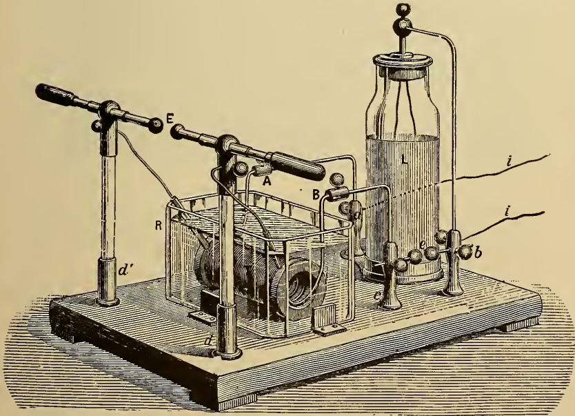
FIG. 4.—Miniature Tesla Apparatus. (E. Ducretet.)
