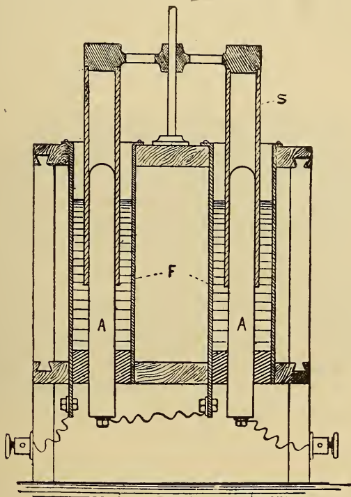
FIG. 32.—Nodon Valve, or Rectifier. (Williams.)
