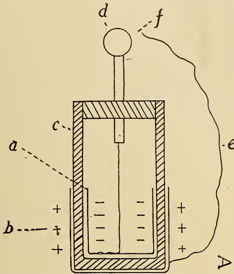
FIG. 23.—Leyden Jar, or Condenser.
